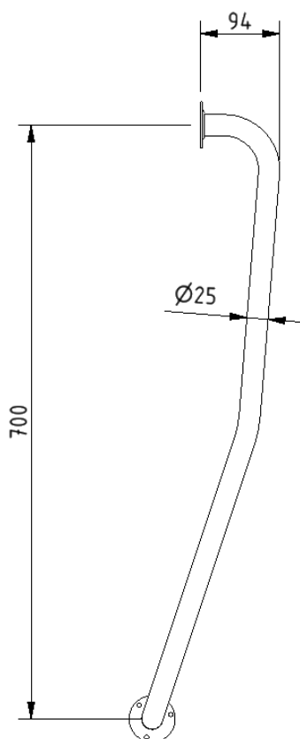
LEFT-HAND
