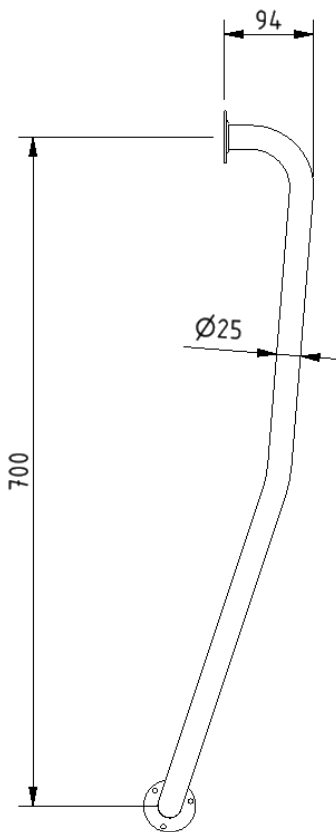
LEFT-HAND
