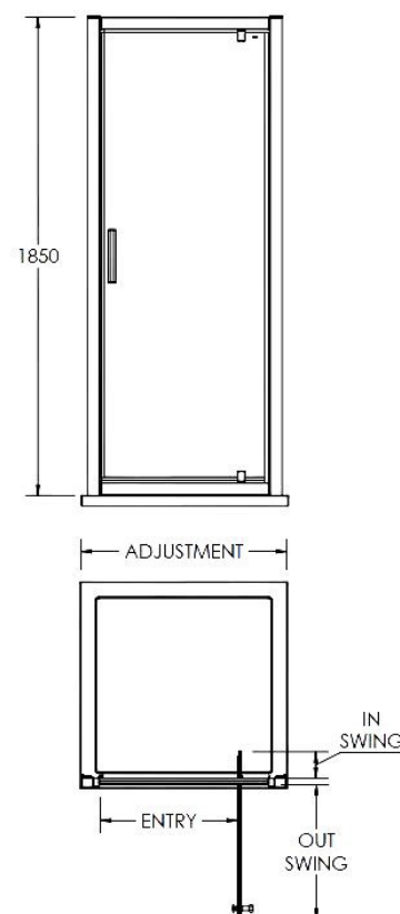
Pacific Pivot Door Enclosure
