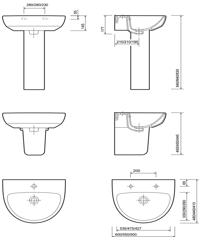
E100 550mm 1TH washbasin on pedestal
