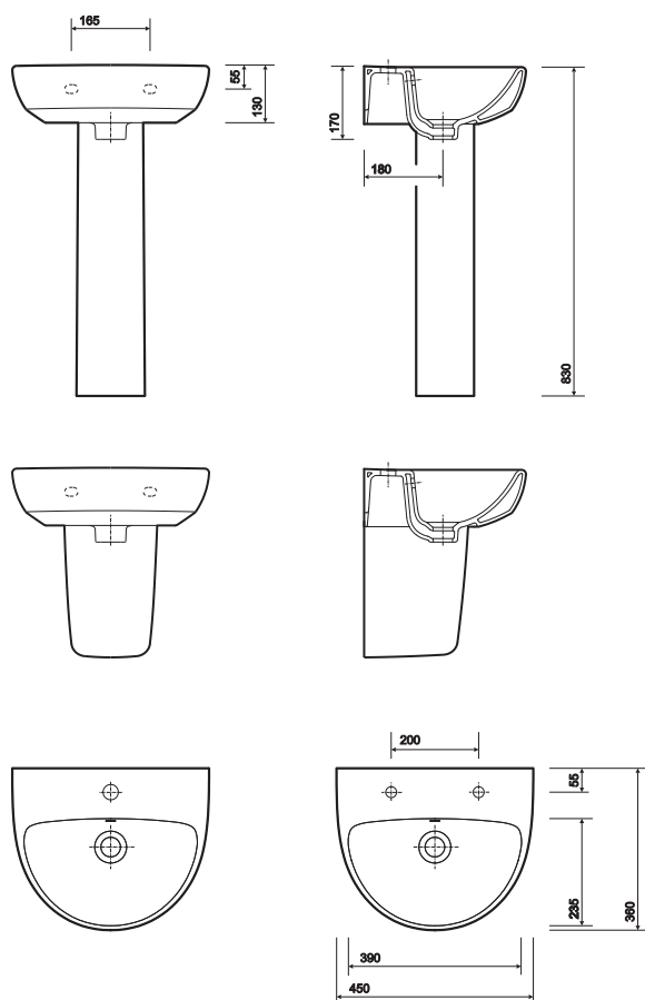
E100 450mm 1TH washbasin on pedestal
