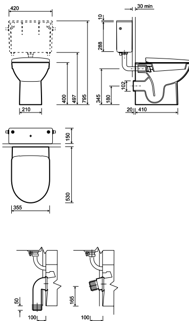
E100 back-to-wall WC suite
