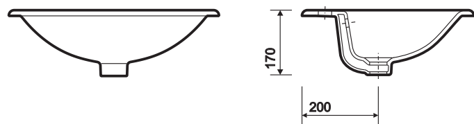
E100 550 1TH countertop basin
